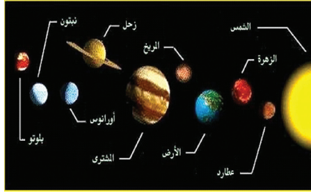
كواكب المجموعة الشمسية
